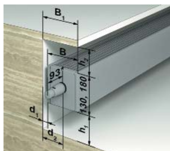
настенный монтаж
