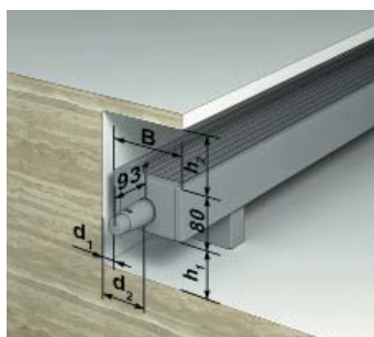
напольный монтаж
