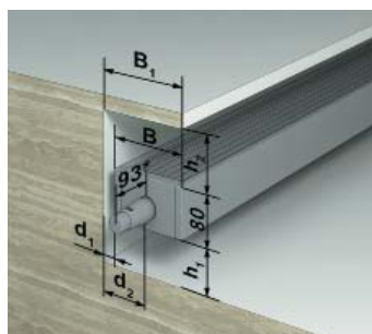
настенный монтаж
