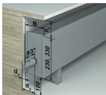
напольный монтаж
